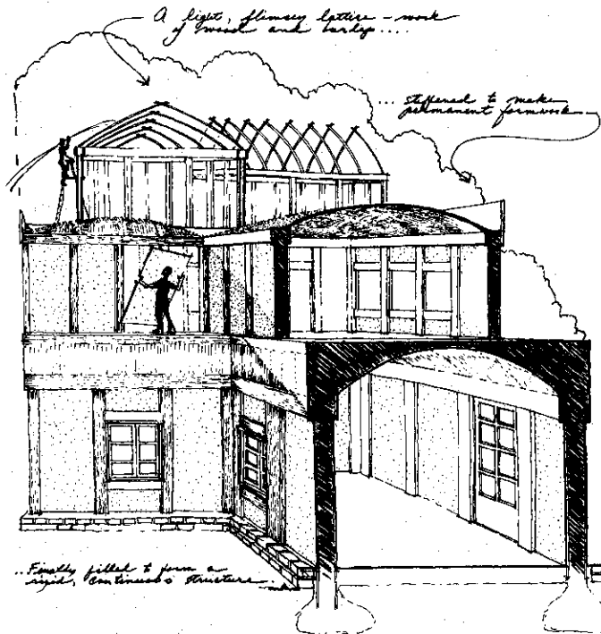
Eine Version von schrittweise erfolgendem Aussteifen, bei der 2½ cm-Dielen, Gipskarton und Sackleinwand als Platten, Leichtbeton als Füllung verwendet werden.
