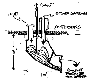
Clivus Kompostgrube.
