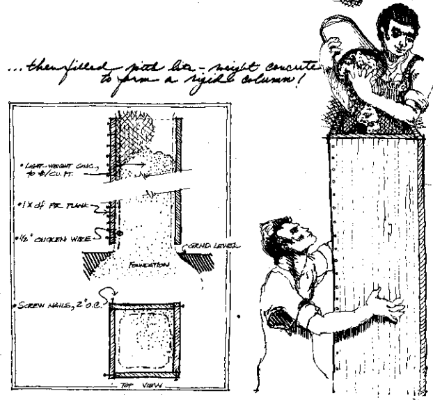
Eine Version von Kastenpfeilern aus 2,5 cm dicken Holzplanken, mit Spiralnutnägeln zusammengenagelt und mit Maschendraht und Leichtbeton gefüllt.
